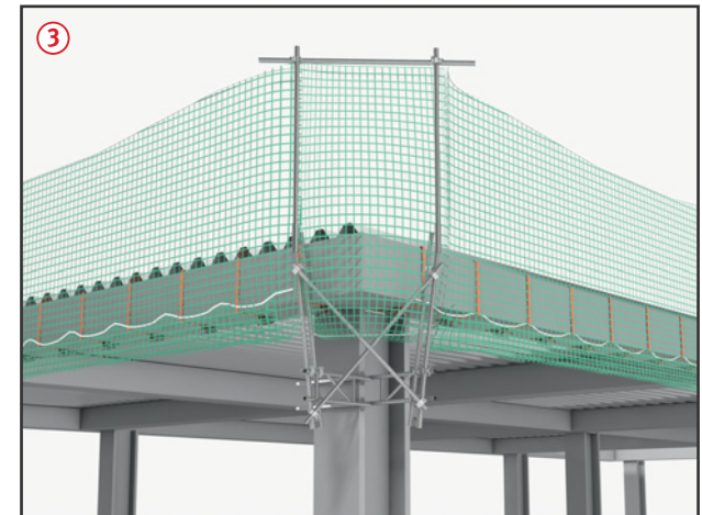
Randsicherung unterhalb der Dachfläche
